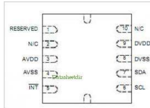
Fig: MEMS IC
